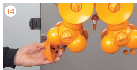
Insertamos las cuñas extractoras. Empujamos las cuñas hasta el fondo para evitar la rotura de las mismas, cuando la máquina esté en funcionamiento.
